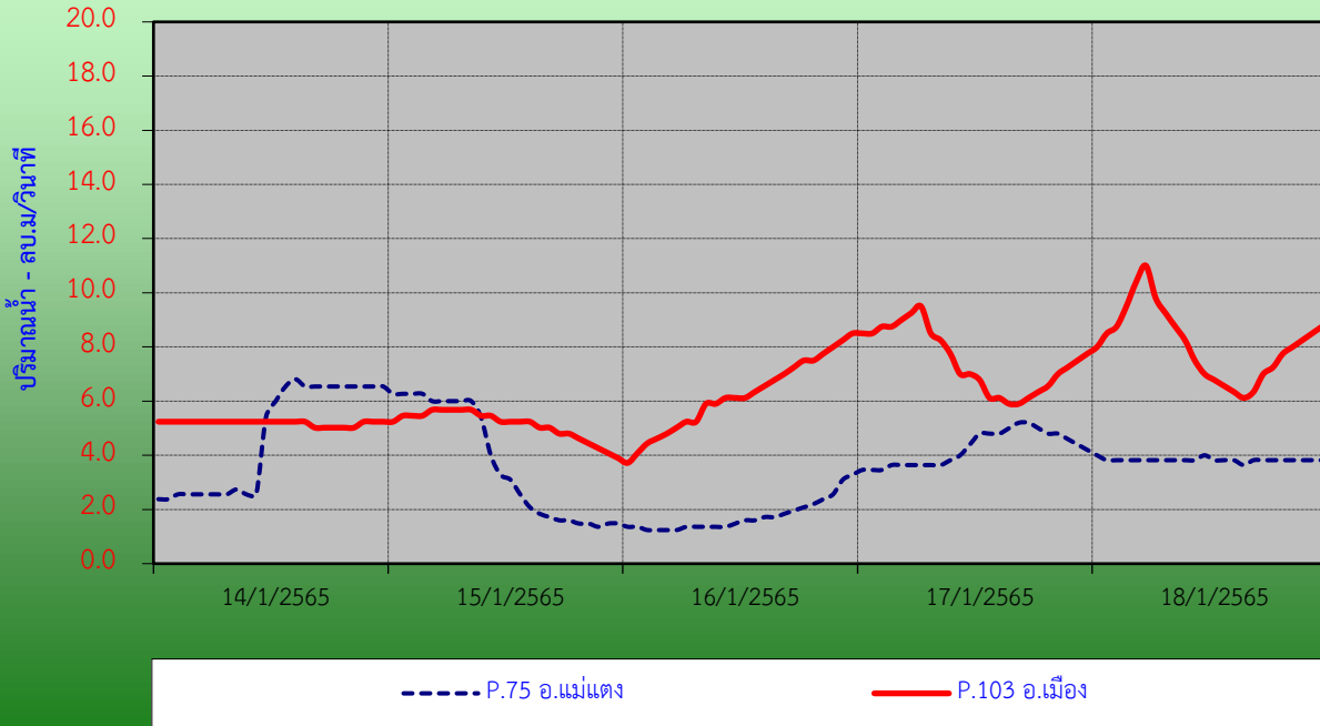
กราฟแสดงปริมาณน้ำปิ้งรายชั่วโมงรอบวันที่ 2/2565 ที่สถานีแม่ น้ำปิ้ง ( P.75) บ้านซ้อแล อ.แม่แตง และที่สถานีแม่ น้ำปิ้ง(P.103) บ้านป่าข่อยใต้ อ.เมือง จ.เชียงใหม่
